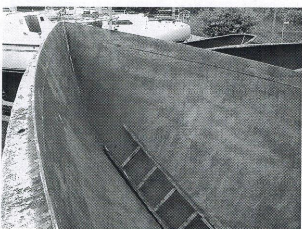
Formens insida.
